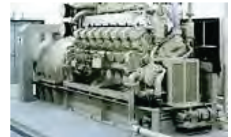
1,000KWクラス ディーゼルエンジン発電設備
